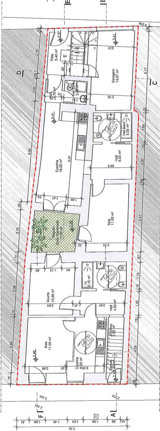
Planta do R/Chão
